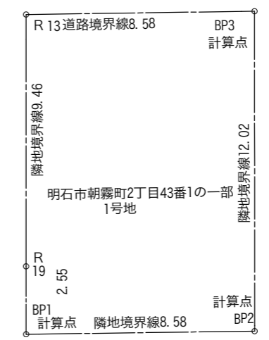
求積表 求積図 S1/200
