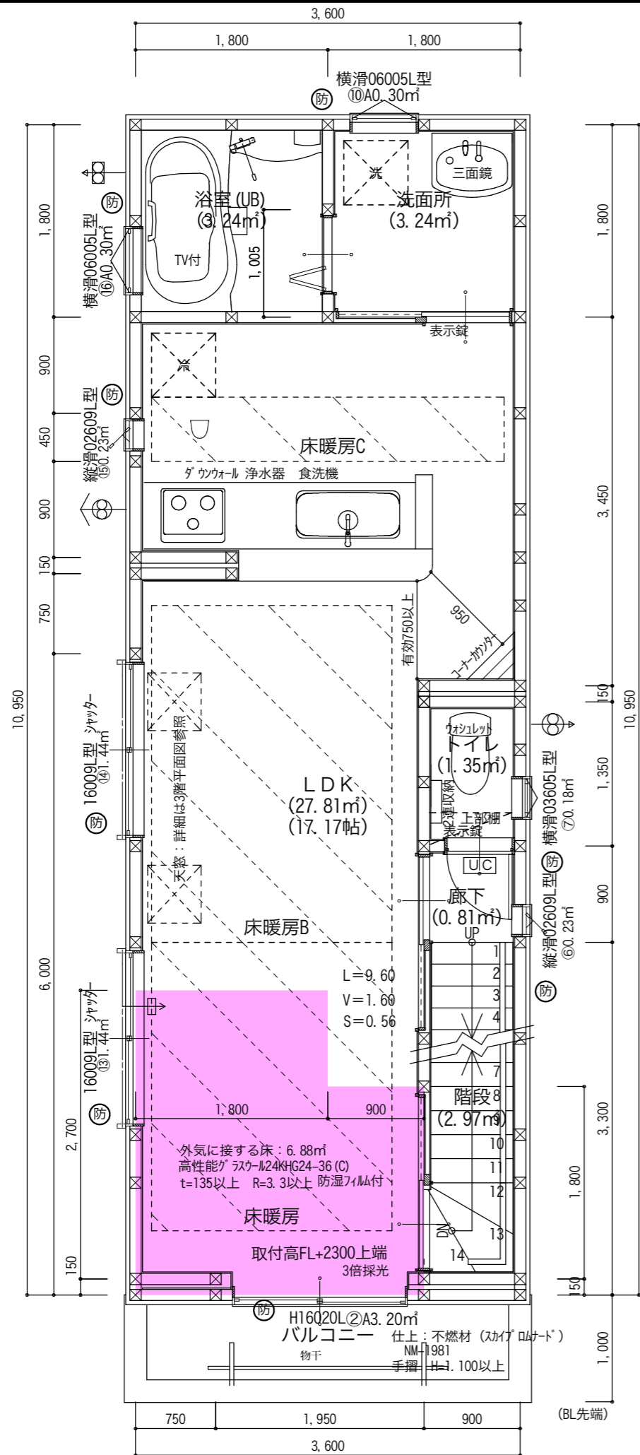
2階 平面詳細図 S:1/50
